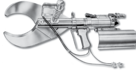
Ürün Kodu | Product Code | كود المنتج : E24 Ayak ve Boynuz Kesme Makası Foot horn Cutting Shear | مقص تقطيع القدم والقرن
