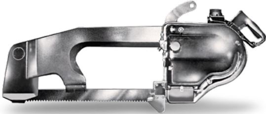
Ürün Kodu | Product Code | كود المنتج : EG02 Karkas Bölme Testeresi (Eksantrik) Carcass Division Saw | منشار تقسيم الذبيحة
